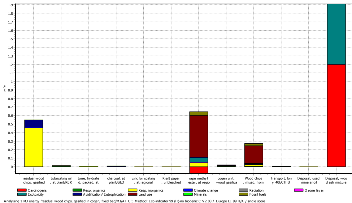
Fig. 6.9 Analyse der Umweltbelastungen der Anlage Güssing pro MJ Holzinput (Eco-indicator 99 (H,A)), Ausbringung der Asche auf Landwirtschaftsfläche
