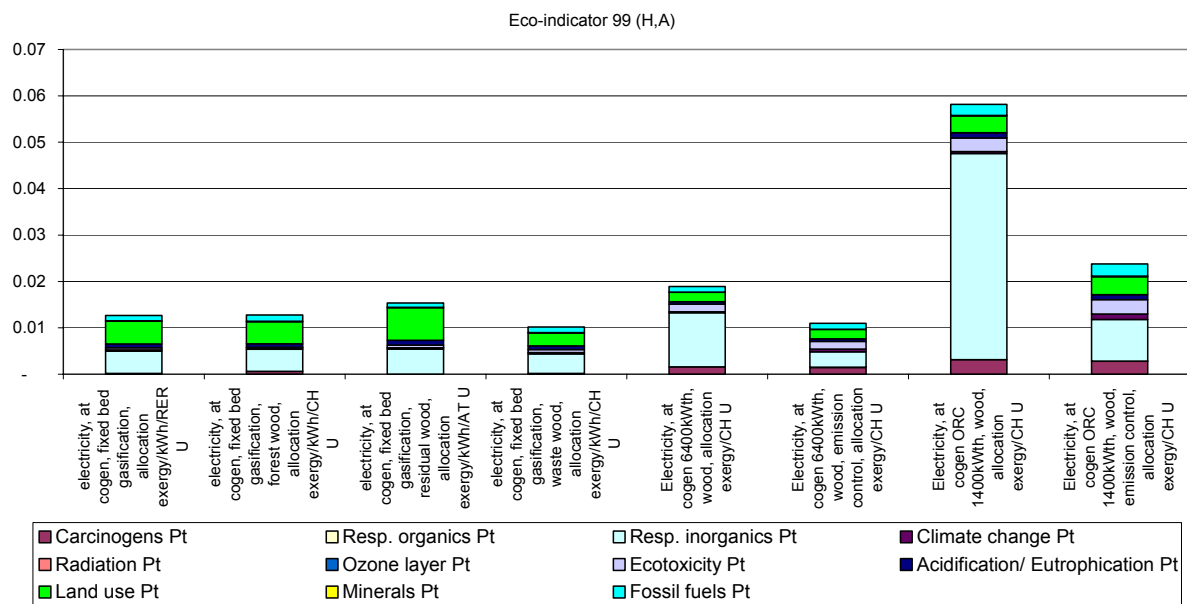
Fig. 6.10 Vergleich der Umweltbelastungen der Holzgas-WKK mit Holzverbrennungs-WKK pro kWh Strom bei Allokation nach Exergie (Eco-indicator 99 (H, A))
