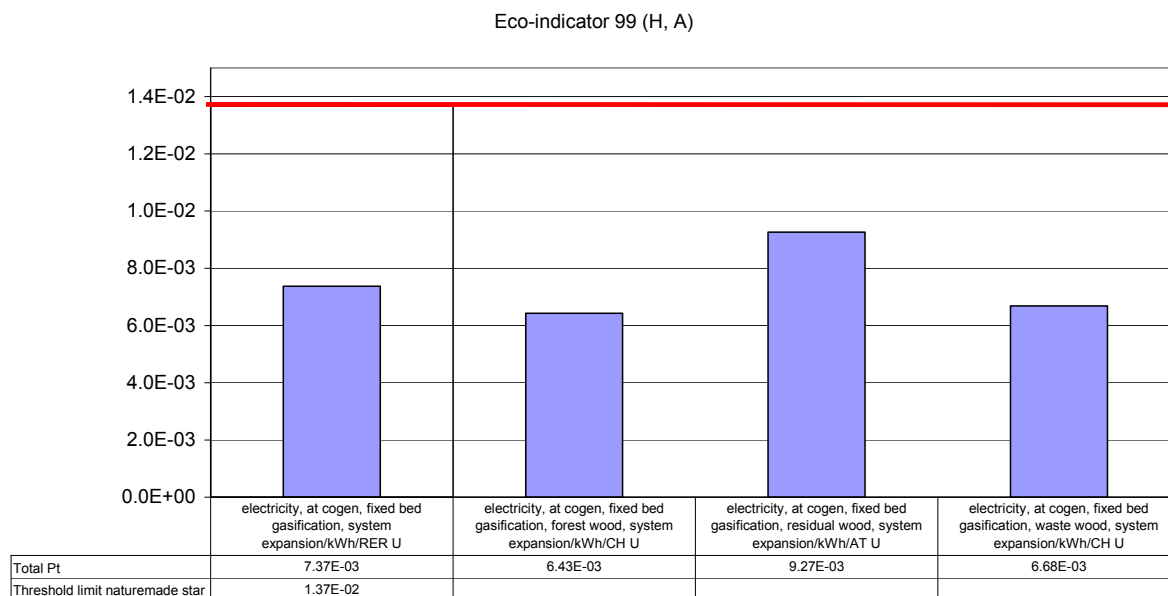
Fig. 6.1 Vergleich der Umweltbelastungen der Holzgas-WKK mit dem Grenzwert für Ökostrom (Eco-indicator 99 (H,A))
