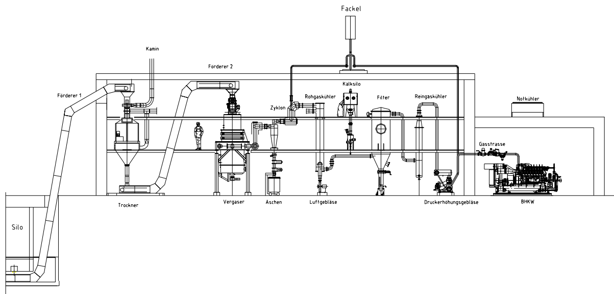
Fig. 4.1 Schematische Darstellung der Holzvergassungs- und WKK-Anlage in Spiez
