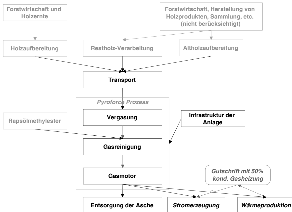
Fig. 2.2 Prozessflussbild der Bereitstellung von Strom aus einer Holzgas-WKK mit Pyroforce-Festbett-Gleichstrom-Vergasung und trockener Gasreinigung
