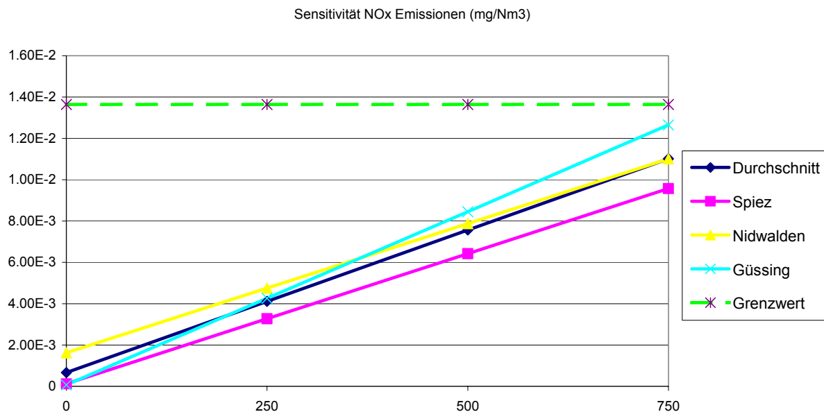
Fig. 6.5 Sensitivitätsanalyse für NO x Emissionen (mg/Nm 3 ), Vergleich der Umweltbelastungen der Holzgas-WKK mit dem Grenzwert für Ökostrom (Eco-indicator 99 (H,A))
